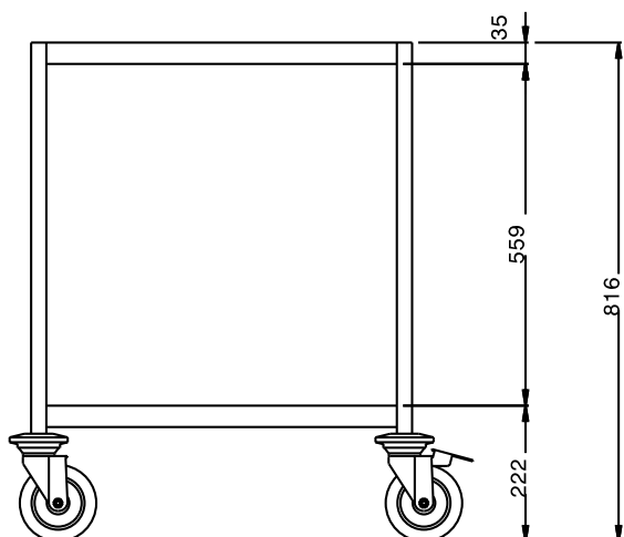
Alzado
